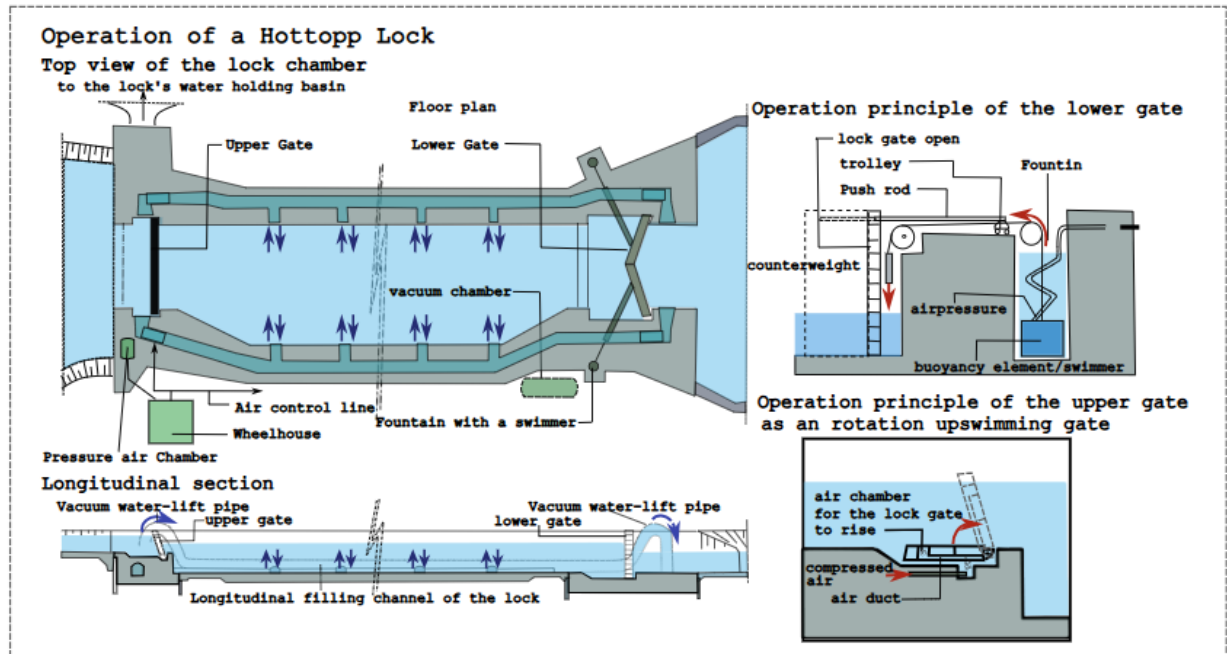
図1：Hotoppの原理・設計に基づく閘門（出典：BAW）
